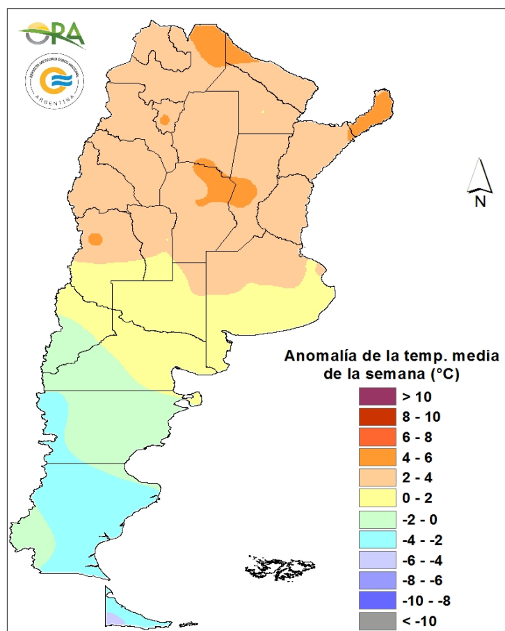
Anomalía de la temperatura media de la semana del 25/09/2024 al 01/10/2024
