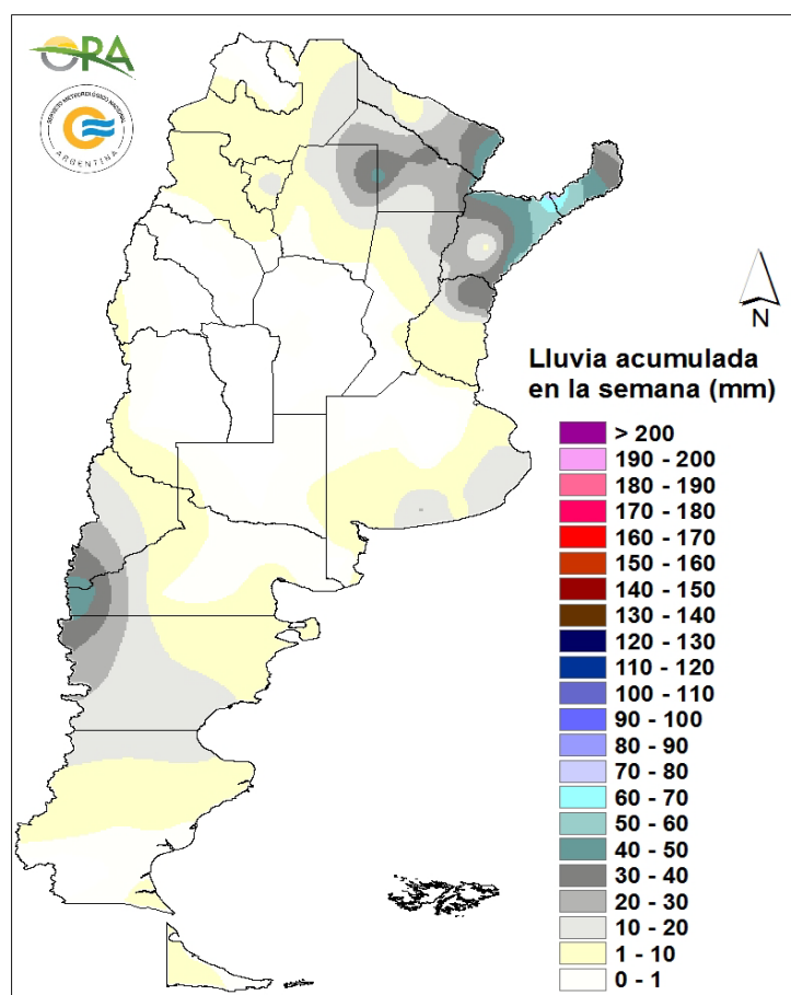
Precipitaciones acumuladas en la semana del 25/09/2024 al 01/10/2024
